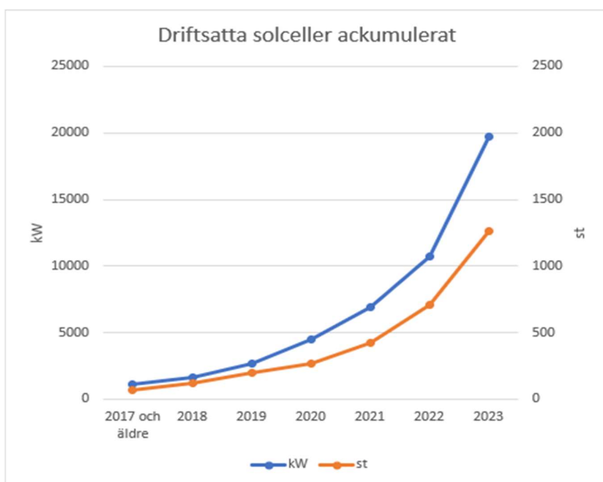
Figur 5 Totala mängden driftsatta solceller sedan start i VEAB:s elnät. Axlarna är angivna i dels installerad effekt men också i antal anläggningar.
